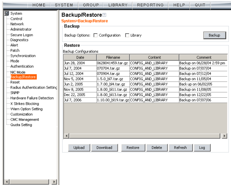
Fig. 2:1-71 Backup/Restore window
